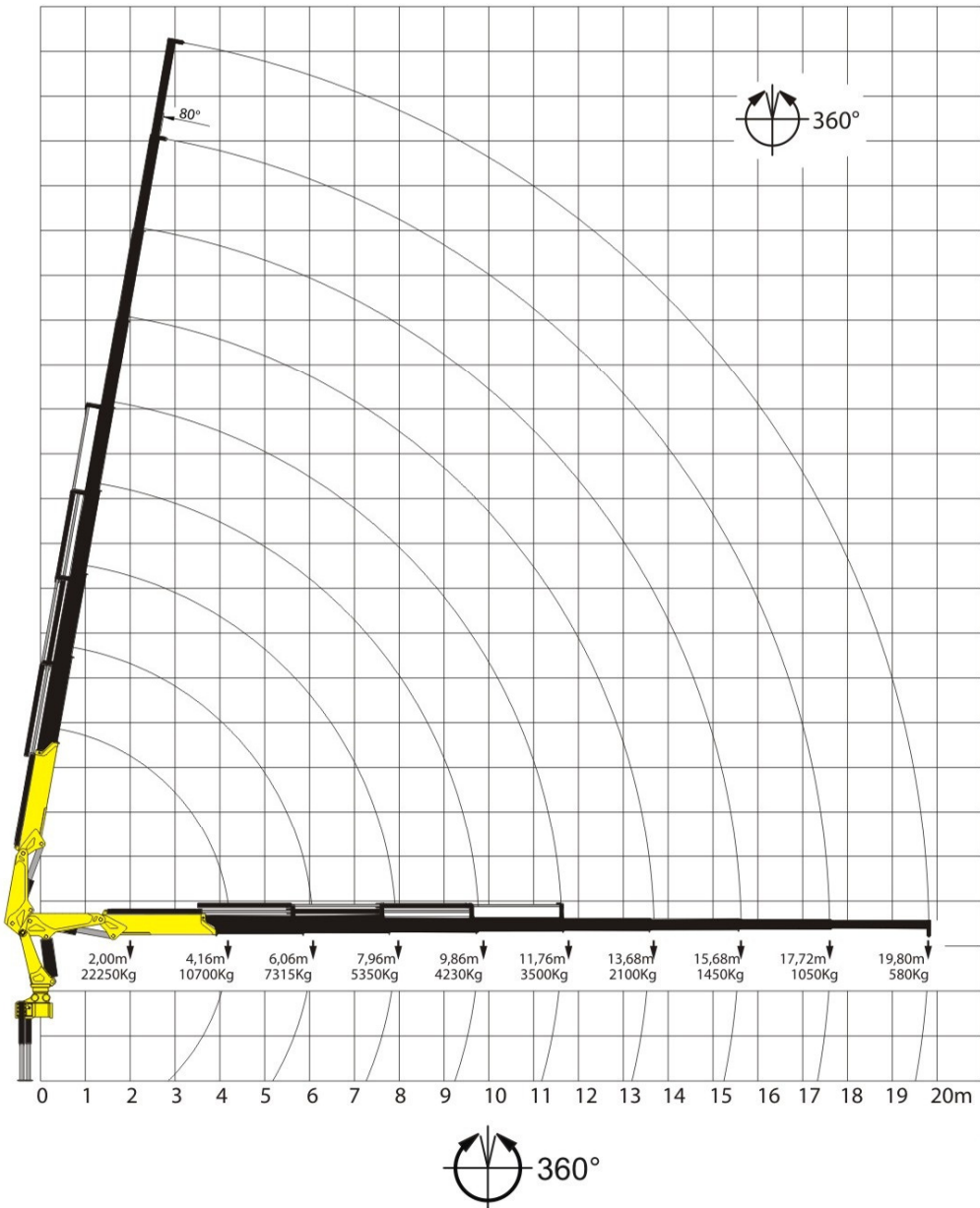
GRÁFICO DE CARGA
