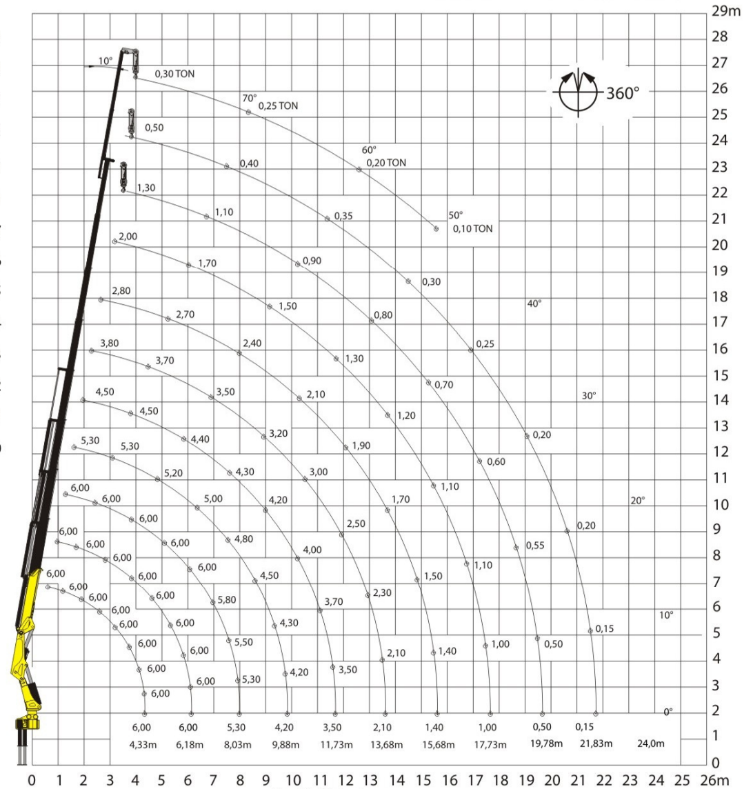
GRÁFICO DE CARGA COM JIB
